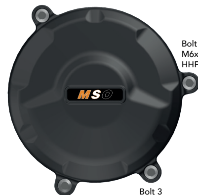
Bolt 4 M6x30 HHF - 8Nm
